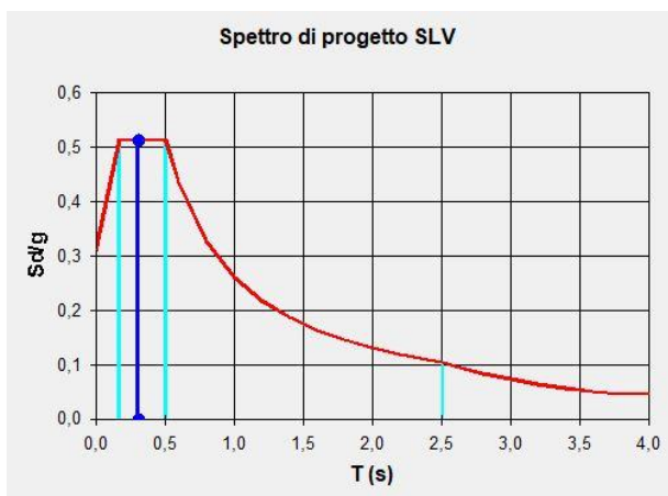
Figura n°5 - Spettro orizzontale di progetto US1 con T_1 = 0,307 s; q = 1,5 .
