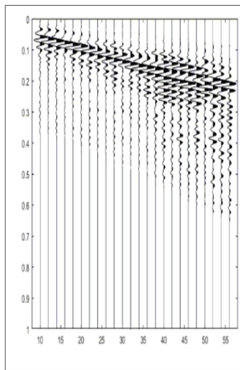
Sismogramma
