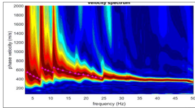
Figura n°6 – Spettro di velocità e curva di dispersione
