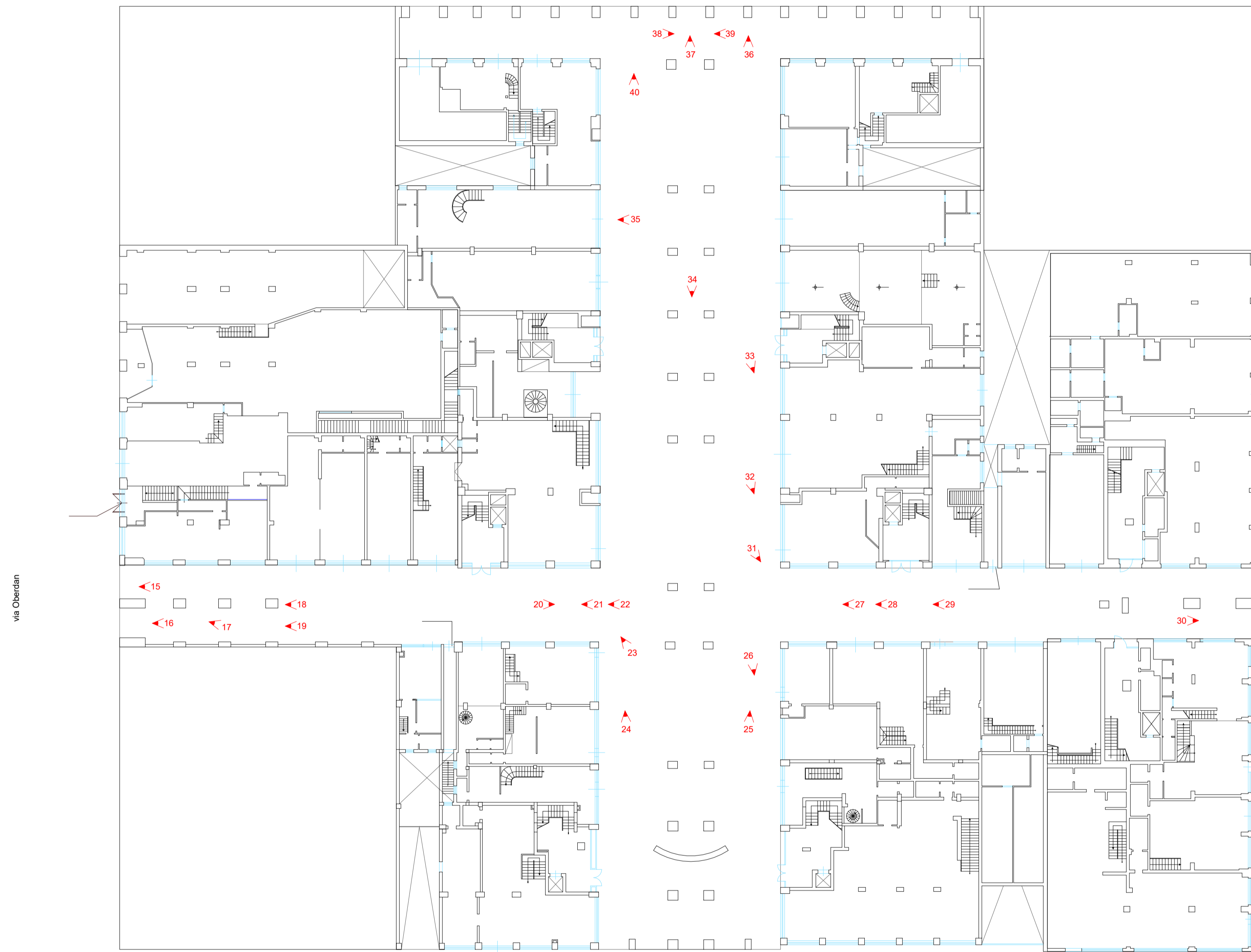
1 0 - Piano Terra - interni A102 1 : 300
