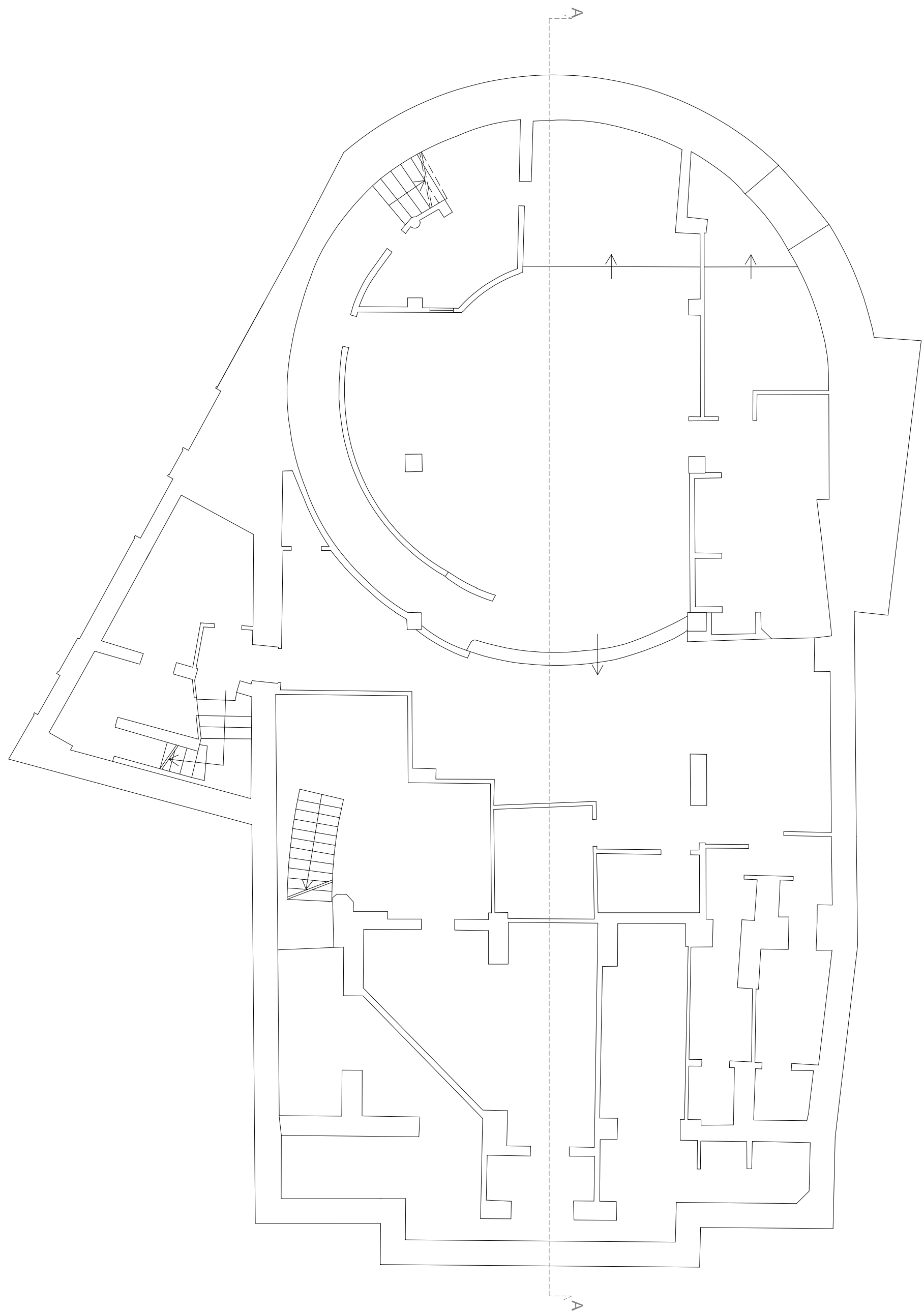
PIANTA PIANO SEMINTERATO
